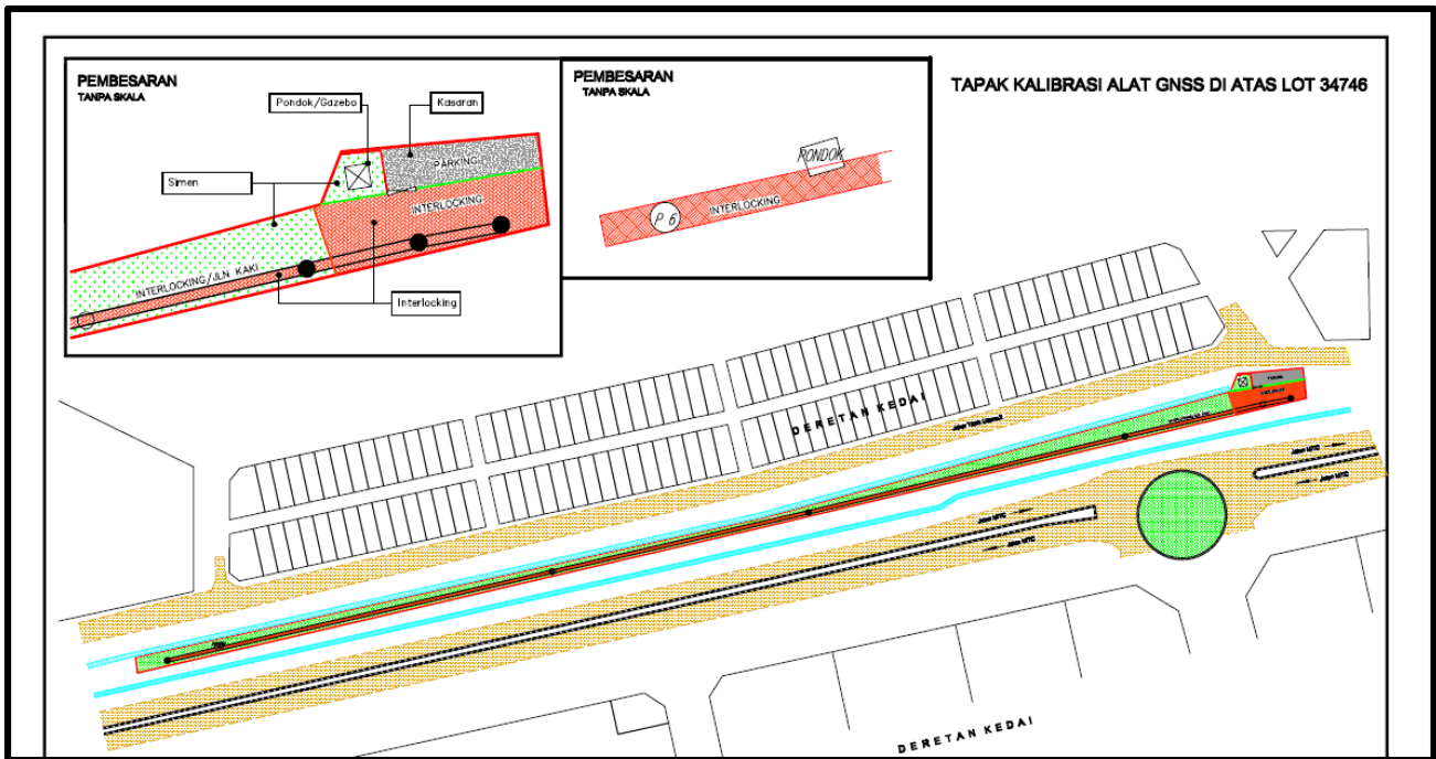
Gambar 2: Pelan tapak kaliberasi GNSS
