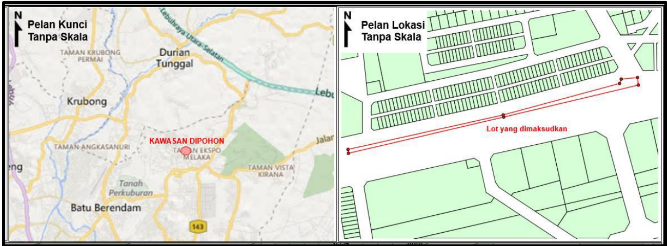
Gambar 1: Pelan kunci dan lokasi tapak kalibrasi
